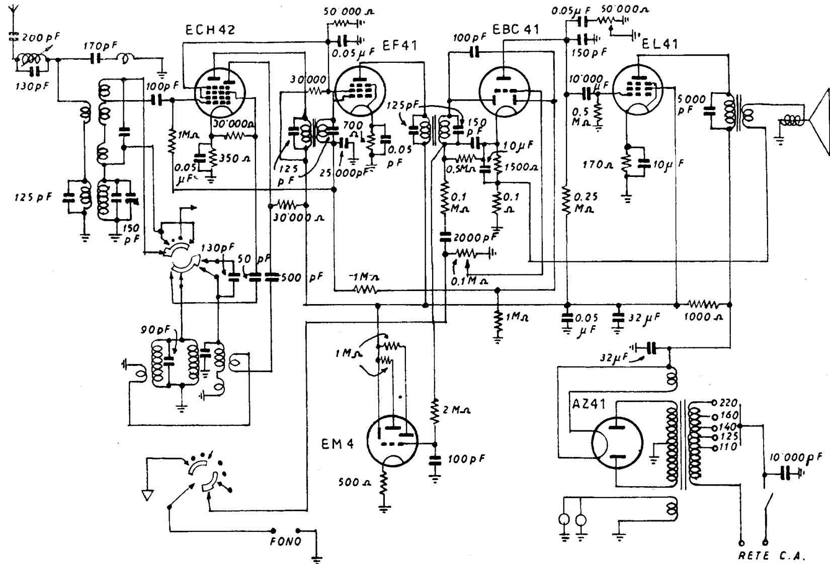
ALLOCCCHIO BACCHINI - Modd. 216 e 226 - Ricevitori con valvole rimlock, provvisti di amplificazione BF con reazione inversa. Media frequenza 465 kc. Potenza d'uscita 3,5 watt indistorti, consumo 54 watt.
